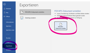
Abbildung 4: Word-Exportieren-Menü.
