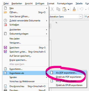
Abbildung 2: Writer-Exportieren-Menü.
